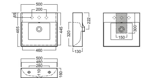
lavabo 50x46,5 washbasin 50x46,5
