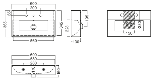
lavabo 60x36,5 washbasin 60x36,5
