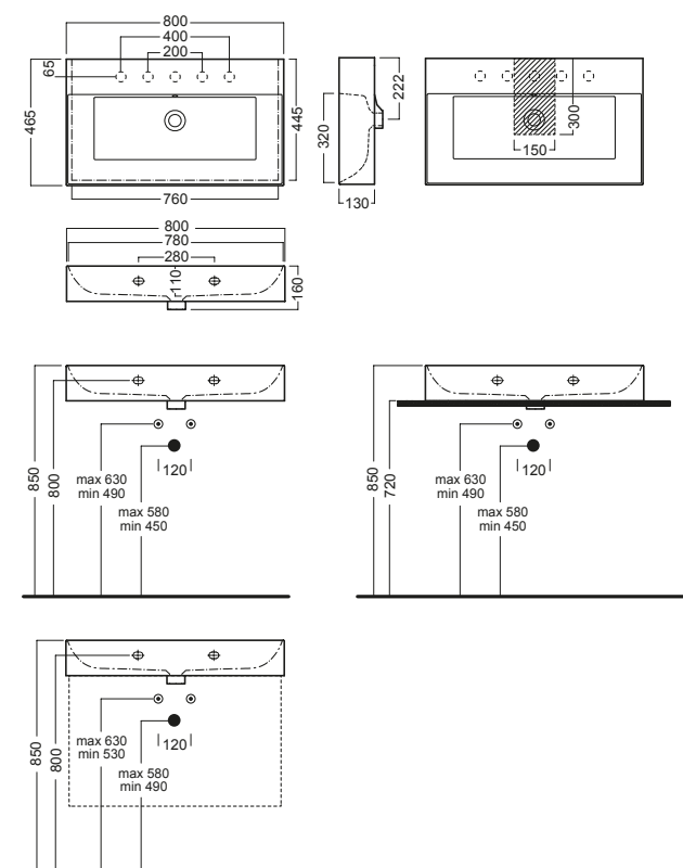
lavabo 80x46,5 washbasin 80x46,5
