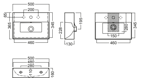
lavabo 50x36,5 washbasin 50x36,5
