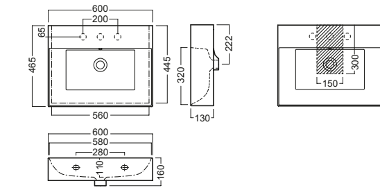
lavabo 60x46,5 washbasin 60x46,5
