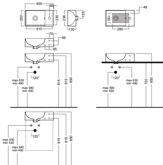
lavamani 45x25 handrinse basins 45x25
